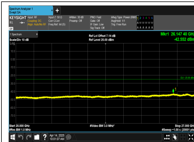
Band7-20MHz-QPSK-21350-100RB#0-20000~27000-PASS
