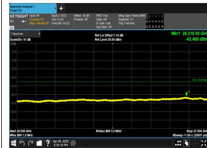
Band7-10MHz-QPSK-20800-1RB#0-20000~27000-PASS
