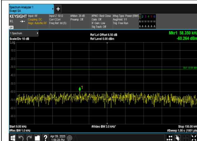
Band5-3MHz-QPSK-20635-1RB#0-0.009~0.15-PASS
