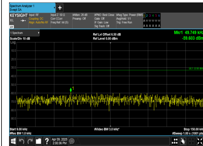
Band5-3MHz-QPSK-20635-15RB#0-0.009~0.15-PASS
