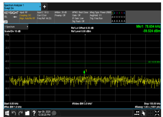
Band4-20MHz-QPSK-20175-1RB#0-0.009~0.15-PASS
