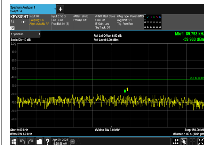
Band4-10MHz-QPSK-20000-50RB#0-0.009~0.15-PASS
