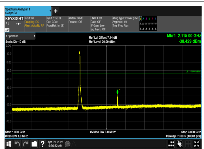
Band4-10MHz-QPSK-20000-50RB#0-1000~3000-PASS
