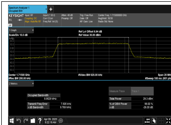
Band4-10MHz-QPSK-20000-50RB#0-PASS
