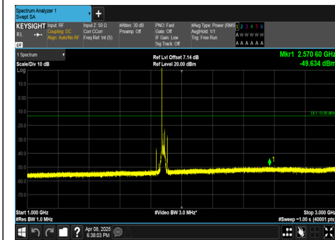
Band2-20MHz-QPSK-18900-1RB#0-1000~3000-PASS
