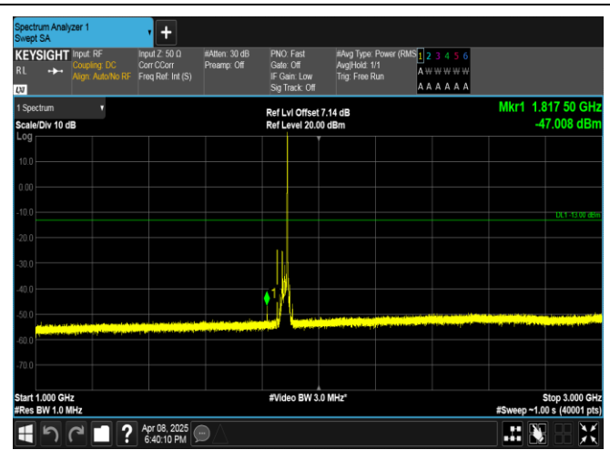
Band2-20MHz-QPSK-18900-1RB#99-1000~3000-PASS
