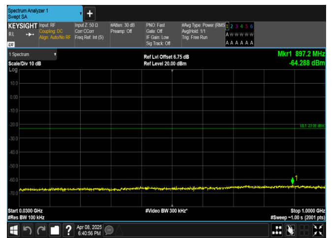
Band2-20MHz-16QAM-18900-1RB#99-30-1000-PASS
