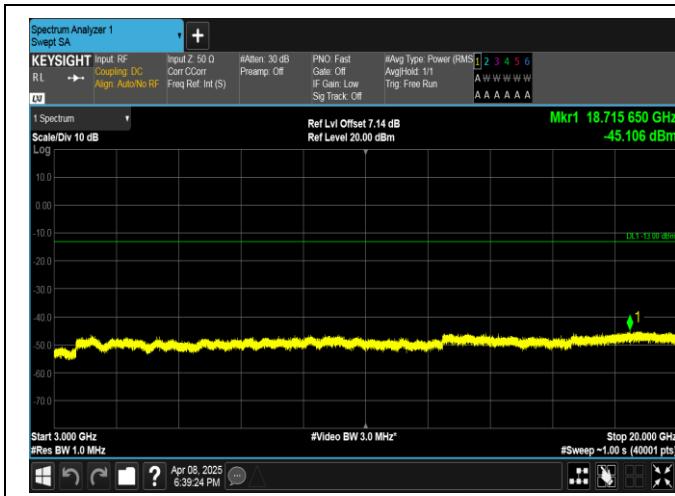
Band2-20MHz-16QAM-18900-1RB#0-3000-20000-PASS
