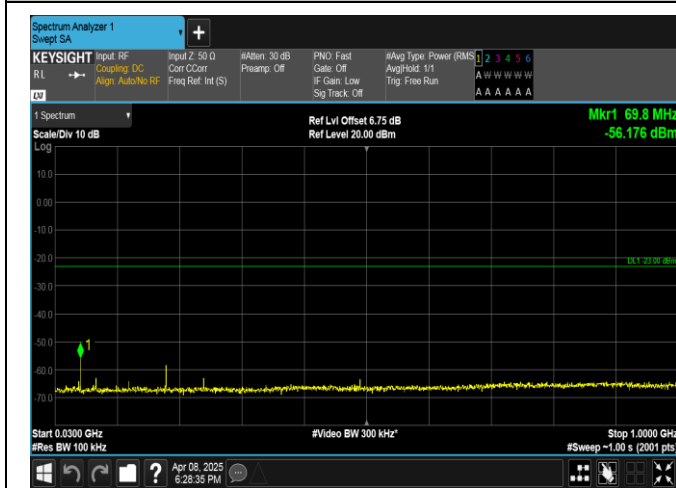
Band2-20MHz-QPSK-18700-1RB#0-30~1000-PASS
