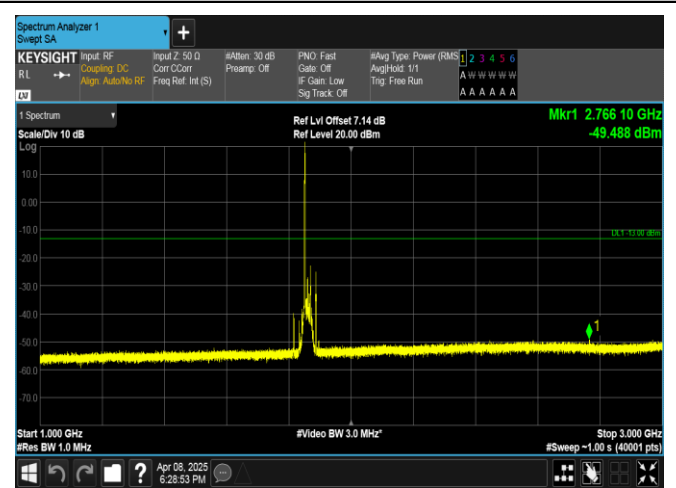
Band2-20MHz-QPSK-18700-1RB#0-1000~3000-PASS
