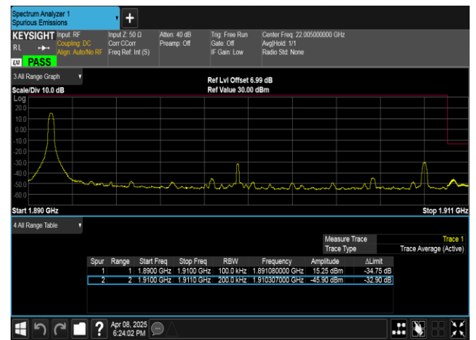
Band2-20MHz-16QAM-18700-1RB#99-PASS
