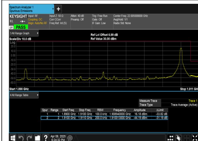
Band2-20MHz-16QAM-19100-1RB#99-PASS
