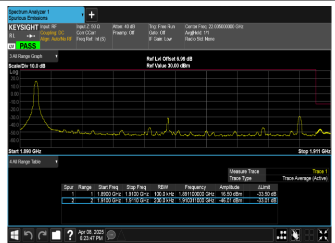
Band2-20MHz-QPSK-18700-1RB#99-PASS
