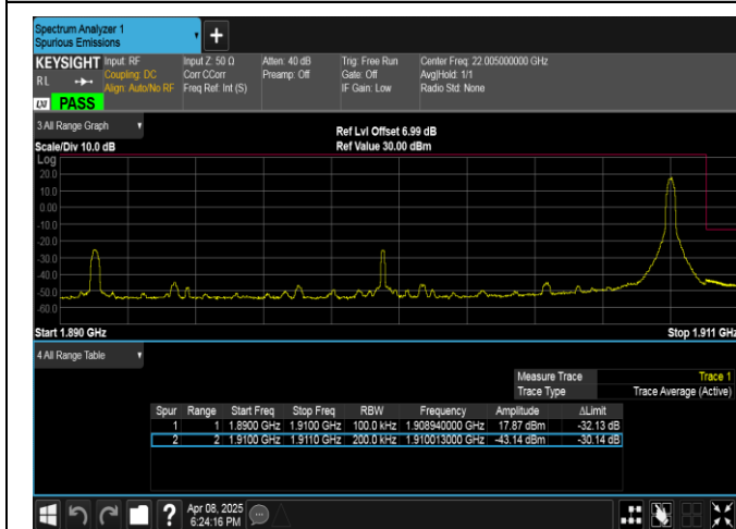
Band2-20MHz-QPSK-19100-1RB#0-PASS
