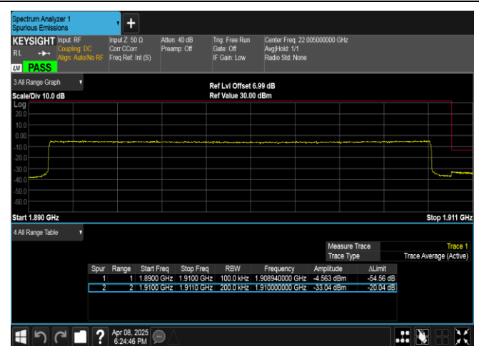
Band2-20MHz-QPSK-19100-1RB#99-PASS
