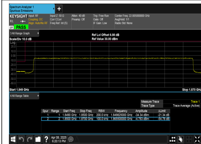
Band2-20MHz-QPSK-18700-100RB#0-PASS
