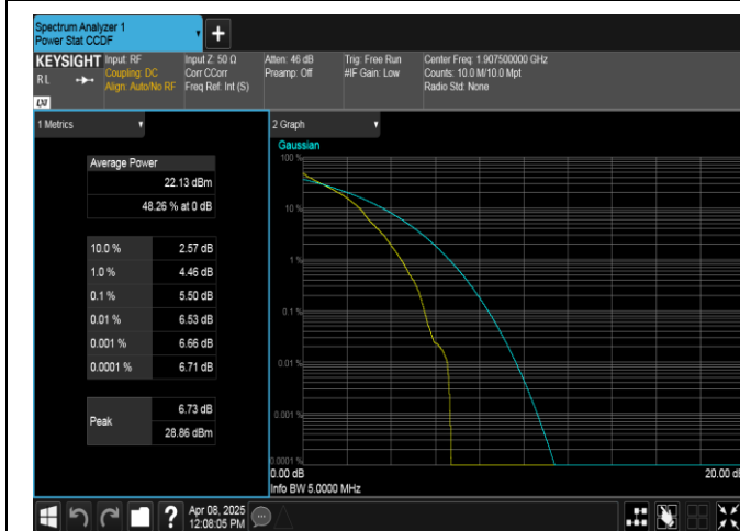
Band2-5MHz-QPSK-19175-1RB#0-PASS
