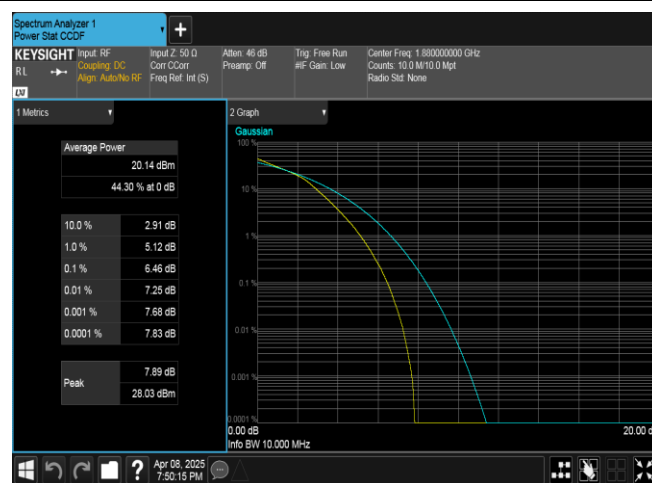
Band2-10MHz-16QAM-18900-50RB#0-PASS
