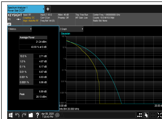
Band2-20MHz-QPSK-18700-1RB#0-PASS
