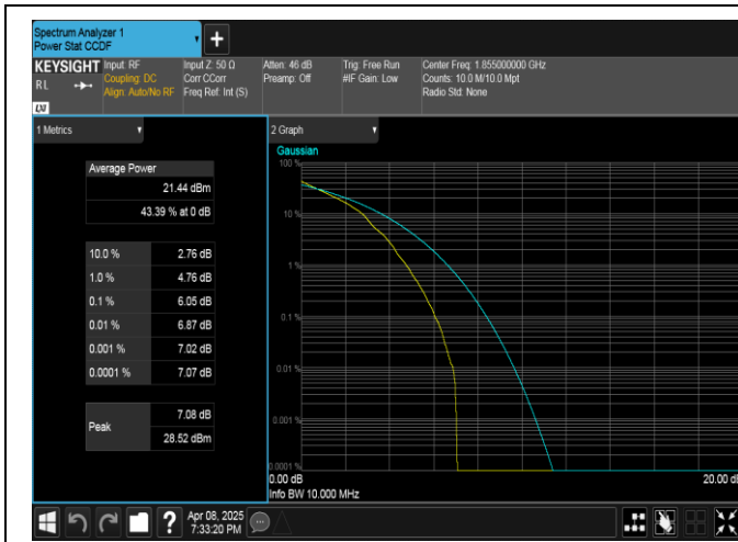
Band2-10MHz-QPSK-18650-1RB#0-PASS
