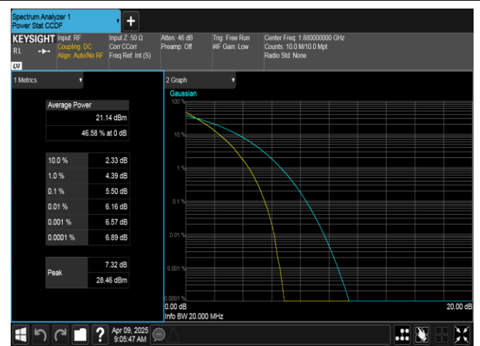
Band2-20MHz-QPSK-18900-100RB#0-PASS
