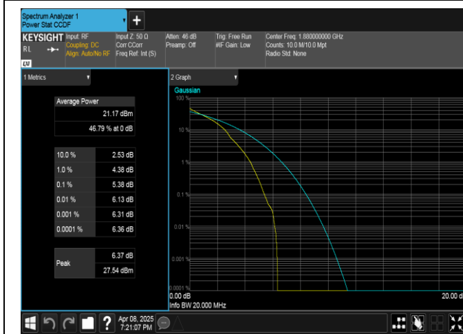
Band2-20MHz-QPSK-18900-1RB#0-PASS
