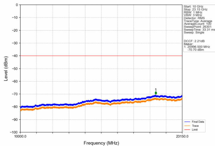
Band40a_10MHz_QPSK_LCH_2310MHz_RB_1_0_NTNV
