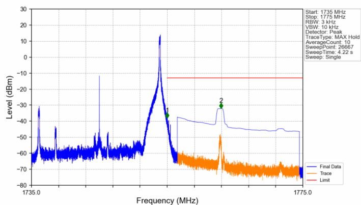
Band4_20MHz_QPSK_HCH_1745MHz_RB_1_99_NTNV
