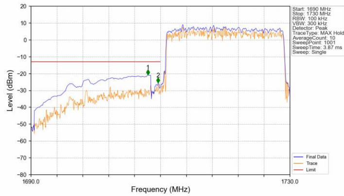
Band4_20MHz_16QAM_LCH_1720MHz_RB_100_0_NTNV
