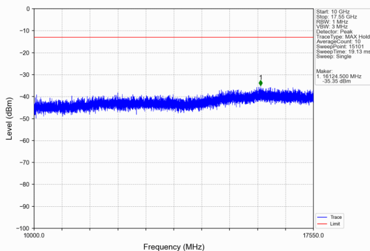
Band4_20MHz_QPSK_HCH_1745MHz_RB_1_99_NTNV
