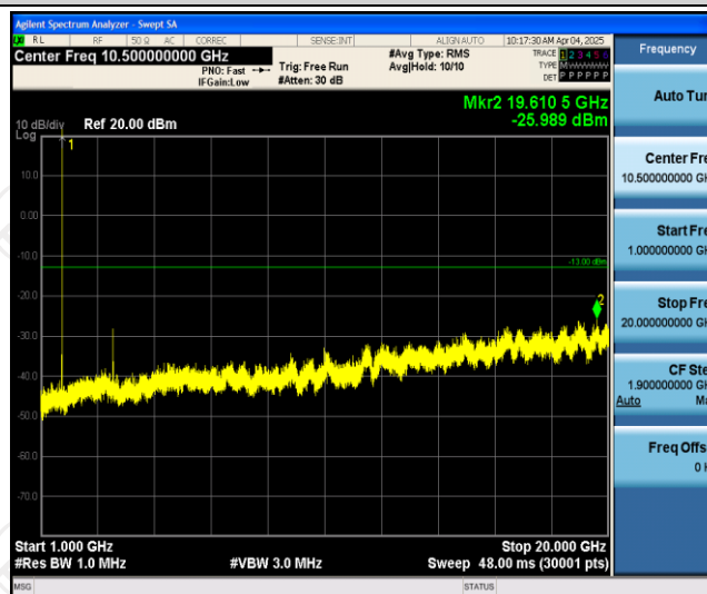
Band4-5MHz-QPSK-19975-1RB#0-Range2:1000~20000MHz
