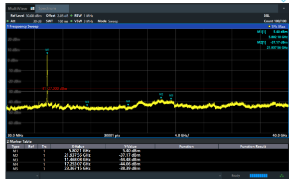
11ac(HT20) CH157
