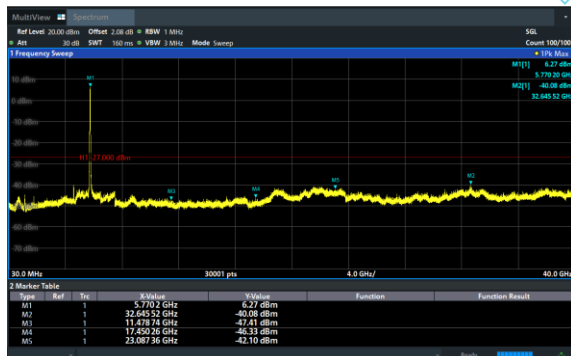
11ax(HE40) CH151
