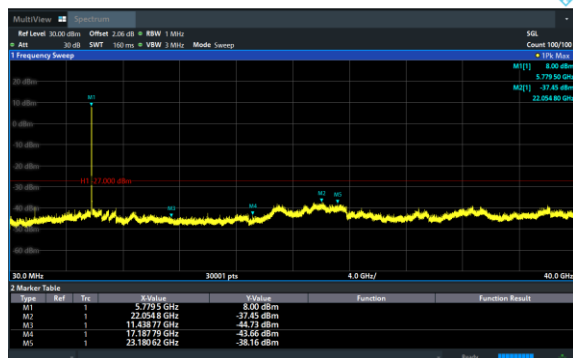
11n(HT20) CH157
