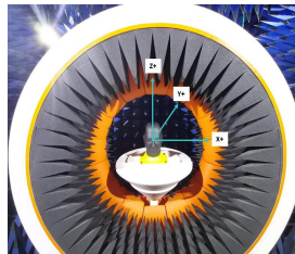
暗室测试坐标轴示意图（头模）
