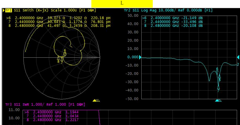
天线阻抗参数测试情况
