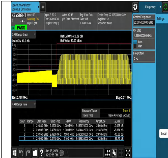
Band41_15MHz_QPSK_39725_75RB#0
