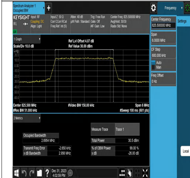
26(824-849)-3MHz-QPSK-26805-15RB#0-PASS
