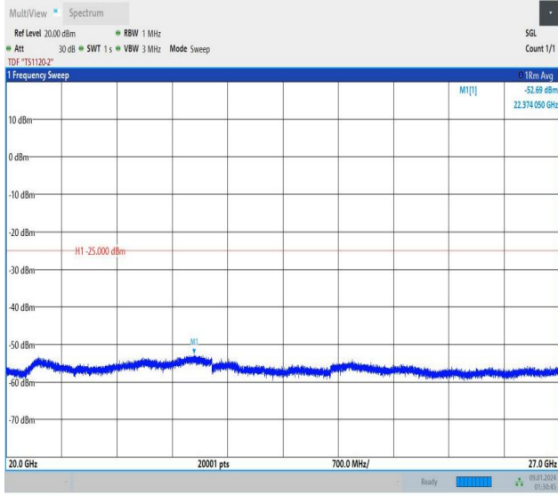
Band7_20MHz_QPSK_20850_1RB#0_20000~27000_20000~27000
