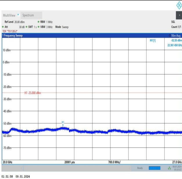
Band7_20MHz_QPSK_20850_1RB#99_20000~27000_20000~27000
