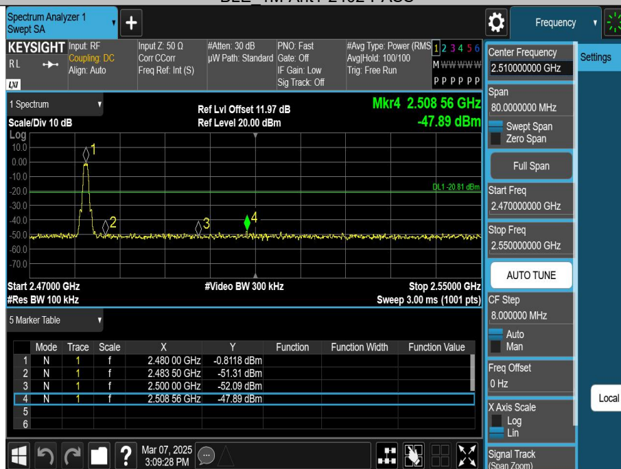
BLE 1M-Ant1-2480-PASS
