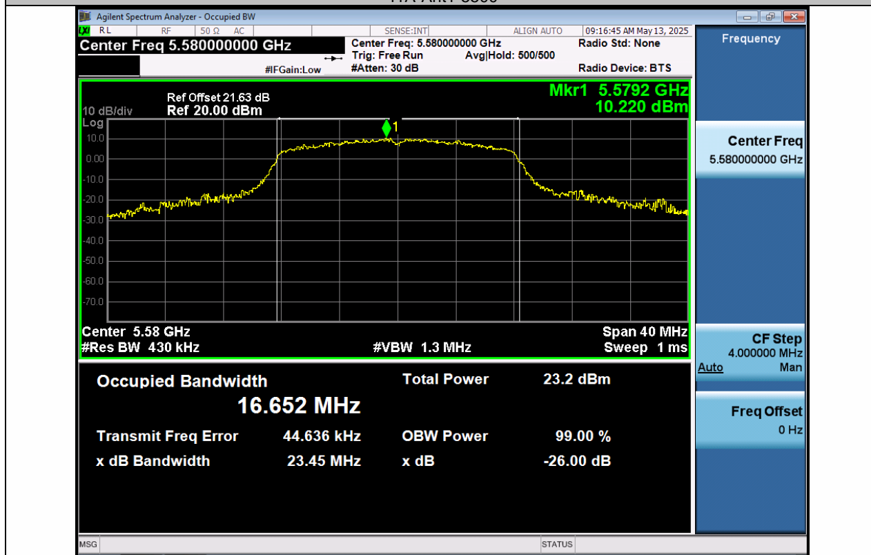
11A-Ant1-5580
