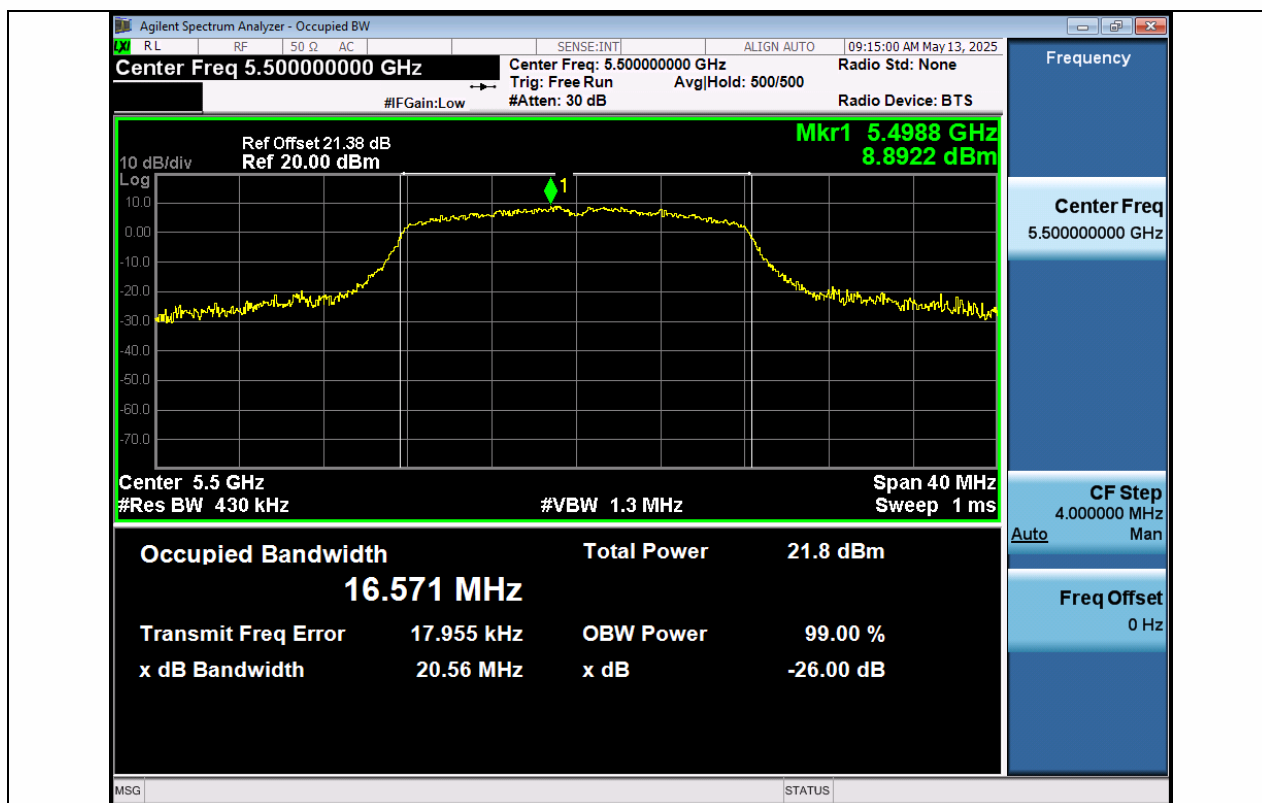
11A-Ant1-5500
