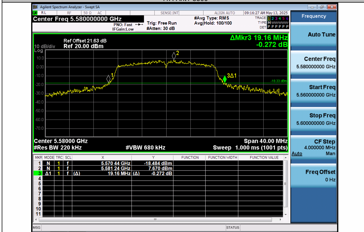
11A-Ant1-5580
