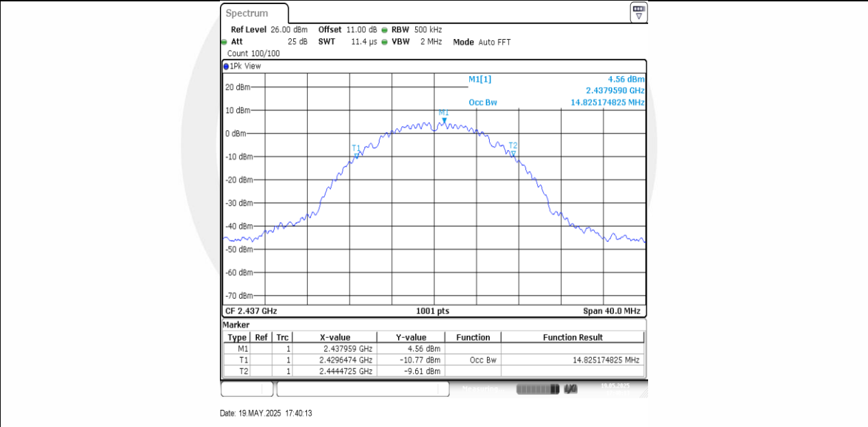
11B-Ant1-2437
