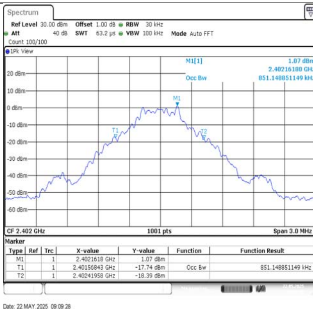
DH5-Ant1-2402
