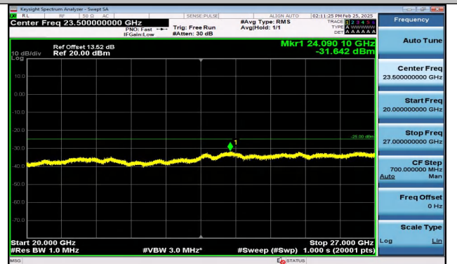
Band41_10MHz_16QAM_41540_1RB#0_20000~27000_2 0000~27000
