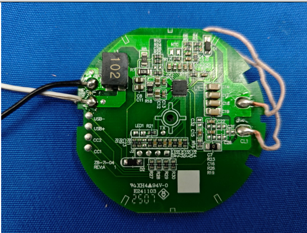
EUT Photo
