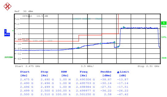
10MHz_Low_QPSK_50@0
