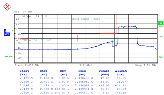
10MHz_Low_16QAM_25@0
