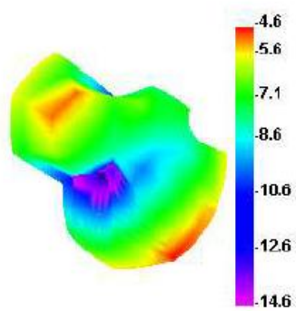
2480.000MHz
