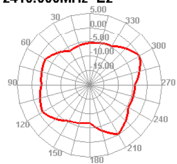
2410.000MHz E2
