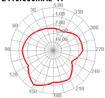
2410.000MHz H
