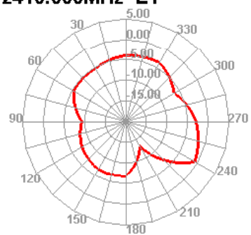
2410.000MHz E1
