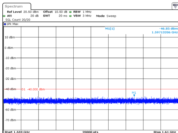
5MHz_Low_QPSK_1@0(1559MHz~1610MHz)
