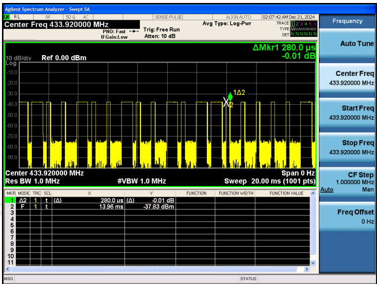
(Time per burst: 0.28 ms*21pcs)
