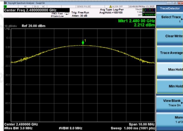
GFSK(CH78)
