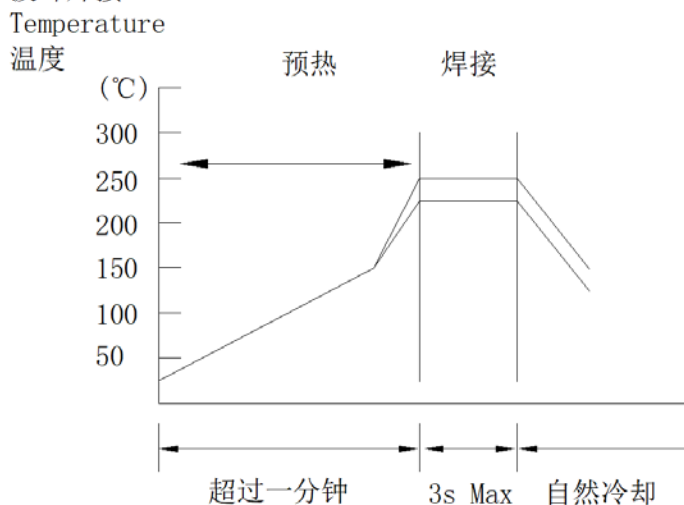
波峰焊接
