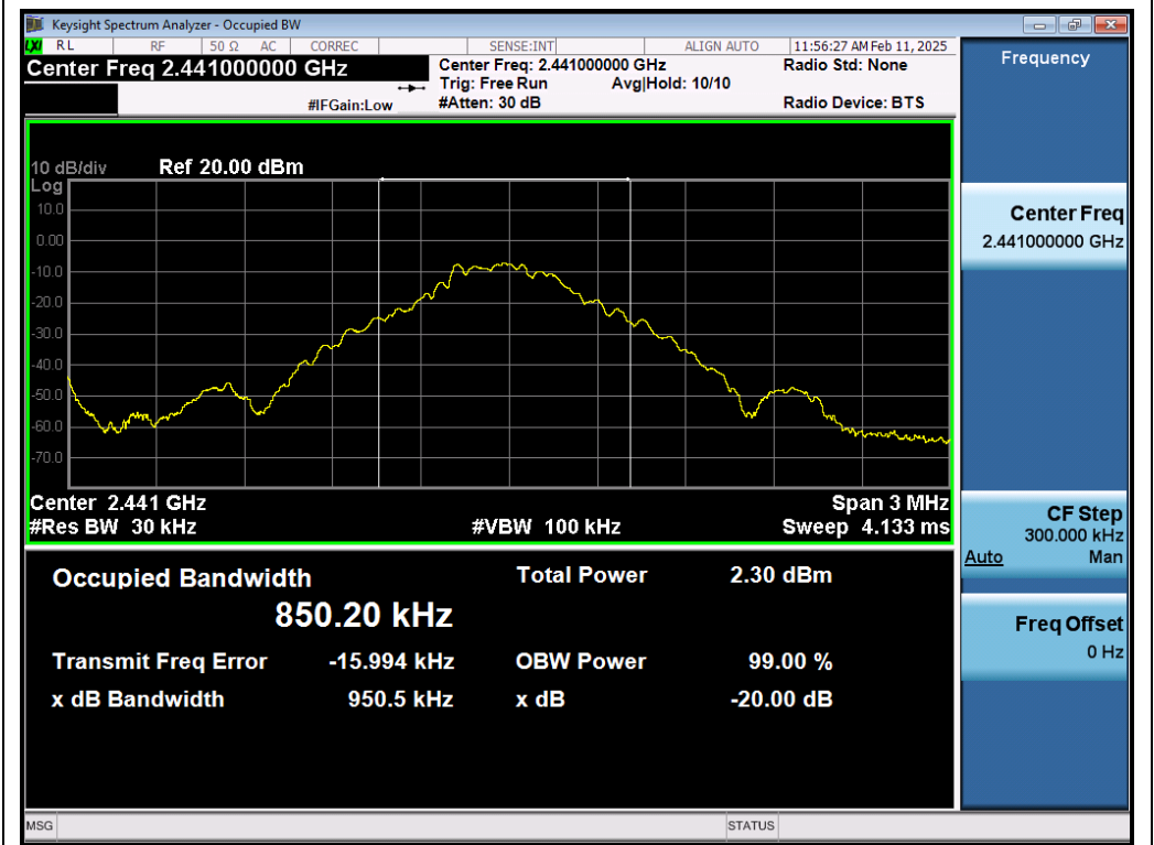
Test_Graph_BR_ANT1_2441_1Mbps_OBW
