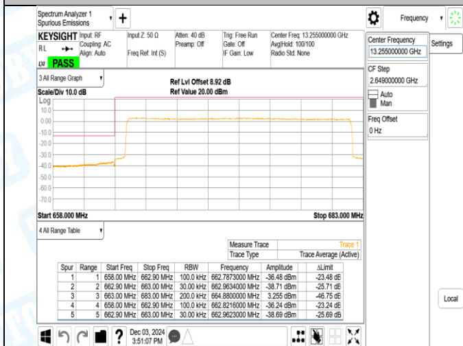
Band71_20MHz_QPSK_133372_1RB#99
