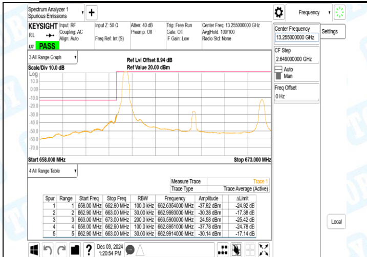
Band71_10MHz_QPSK_133172_50RB#0
