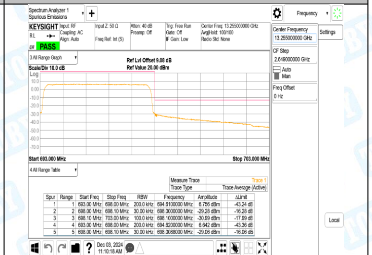
Band71_10MHz_QPSK_133172_1RB#49
