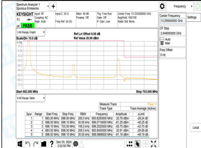
Band71_20MHz_QPSK_133222_1RB#0
