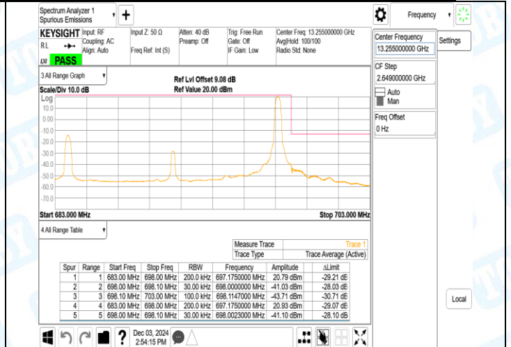
Band71_20MHz_QPSK_133222_1RB#99
