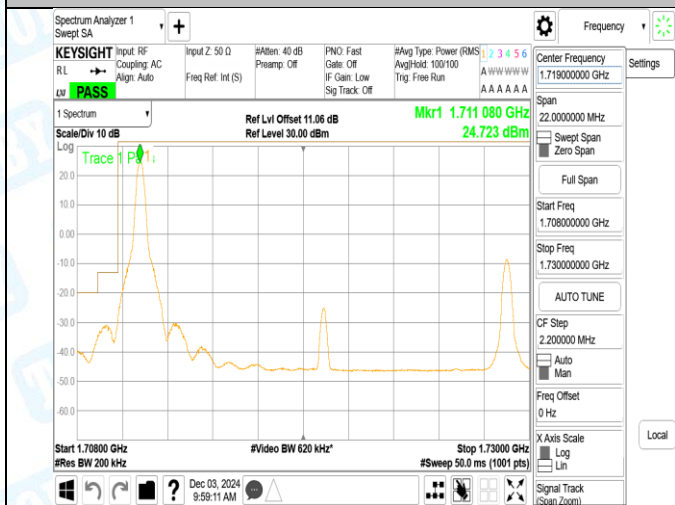
Band66_20MHz_QPSK_132072_100RB#0
