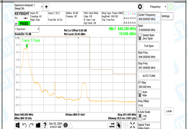
Band5_3MHz_16QAM_20635_15RB#0
