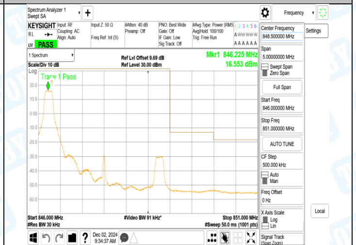
Band5_3MHz_QPSK_20635_15RB#0
