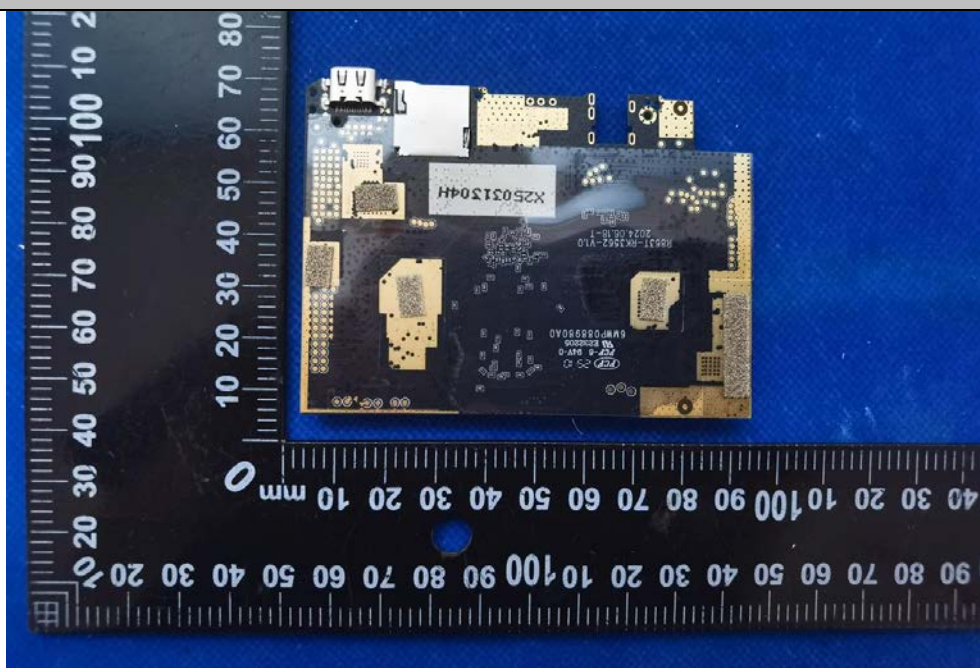
EUT Photo
