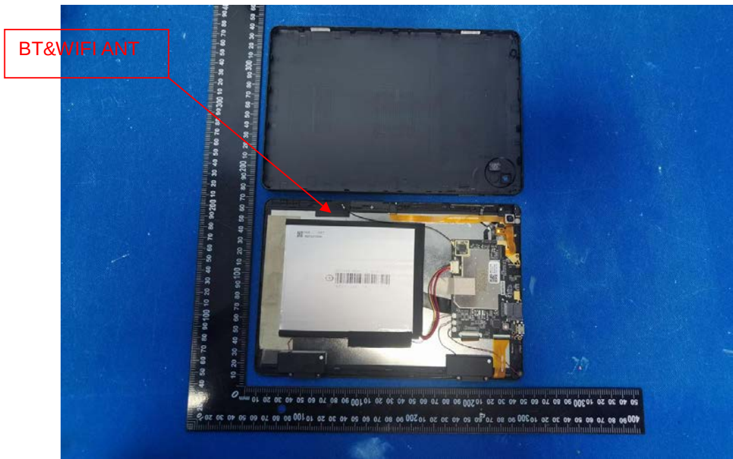
EUT Photo
