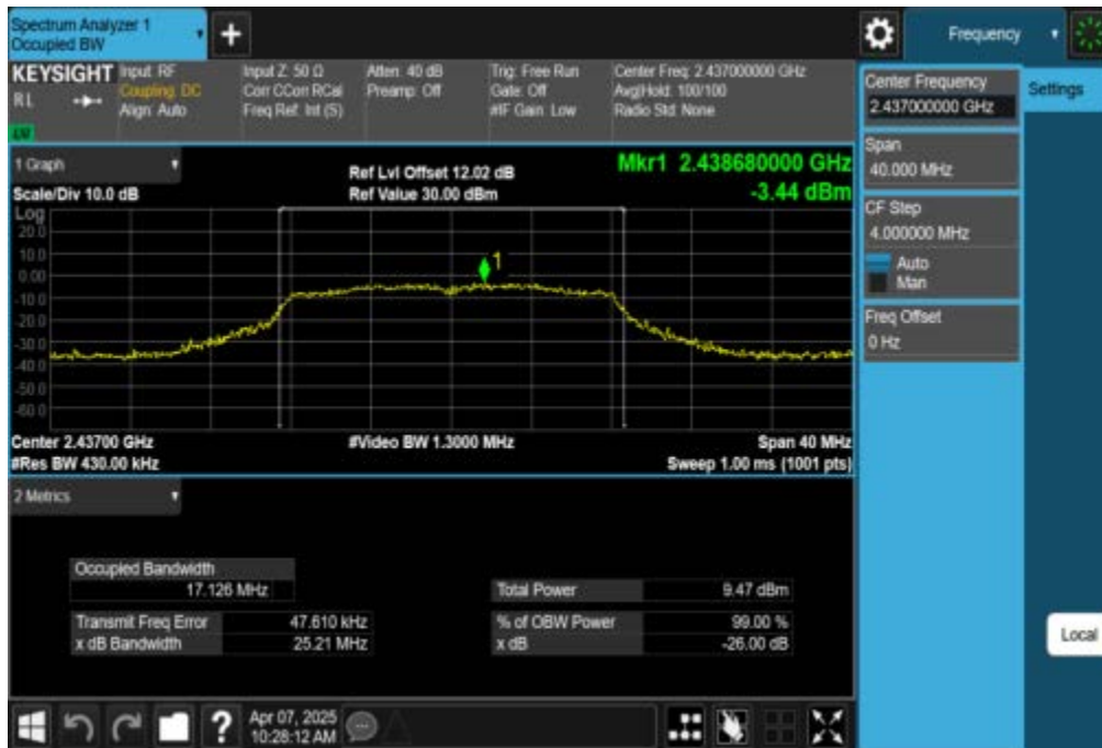
11G-Ant1-2437
