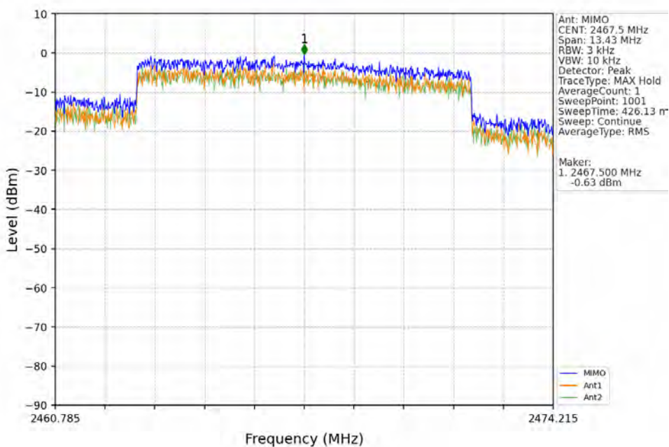
10M_HCH_2467.5MHz_MIMO_NTNV
