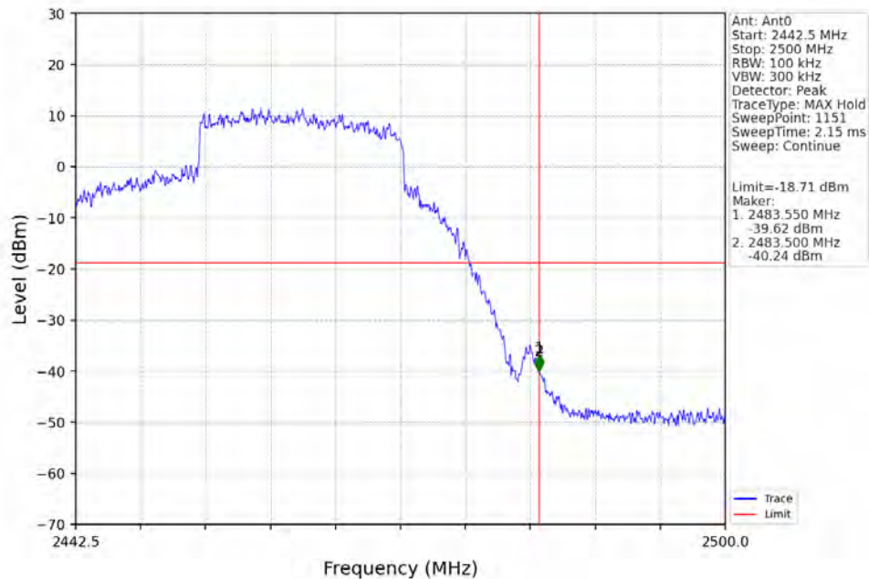
20M_HCH_2462.5MHz_Ant0_NTNV
