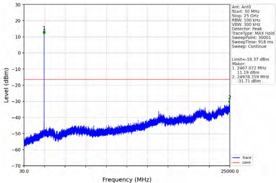
3M_HCH_2468.2MHz_Ant0_NTNV
