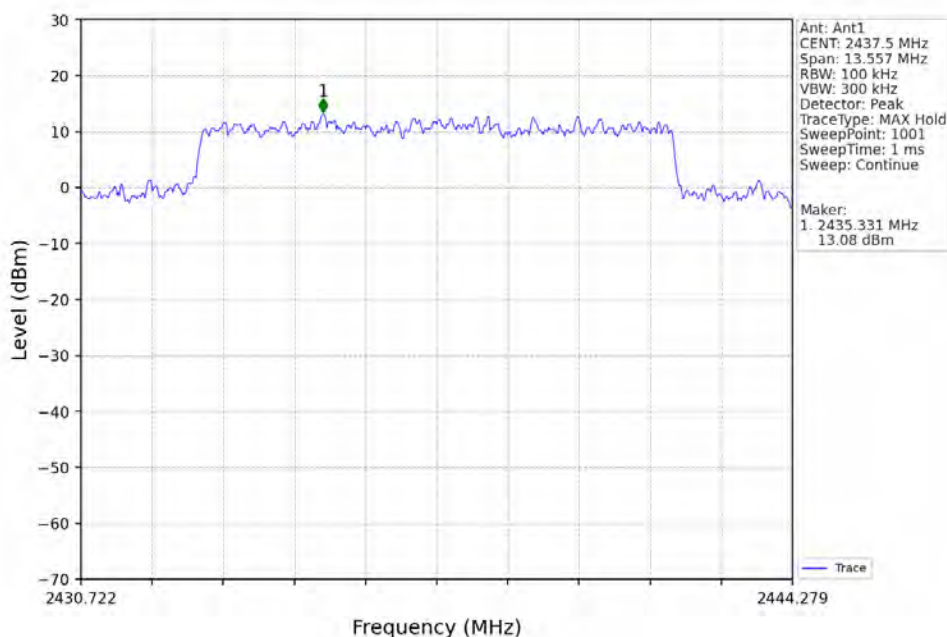
10M_MCH_2437.5MHz_Ant1_NTNV
