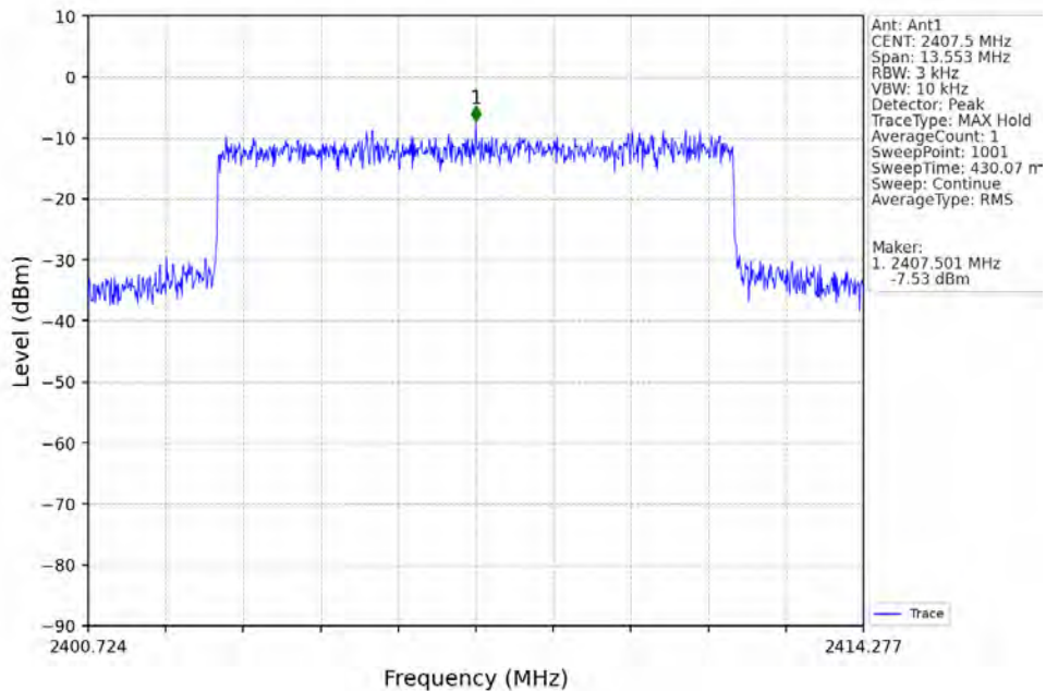
10M_LCH_2407.5MHz_MIMO_NTNV
