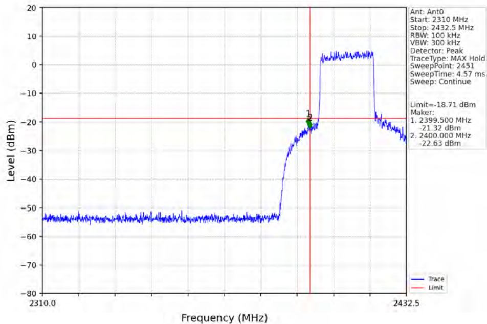
20M_LCH_2412.5MHz_Ant0_NTNV
