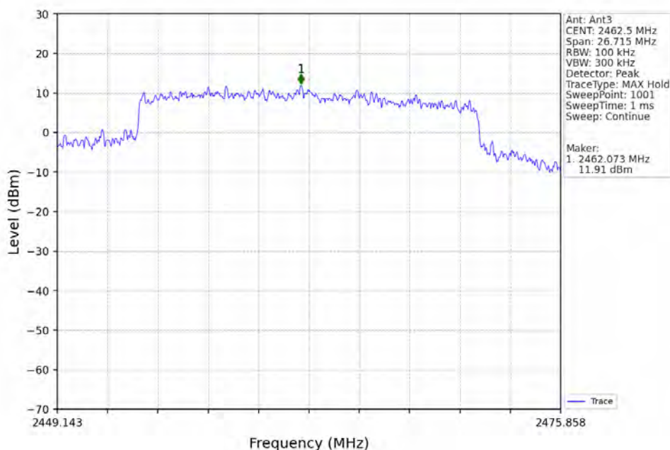
20M_HCH_2462.5MHz_Ant3_NTNV
