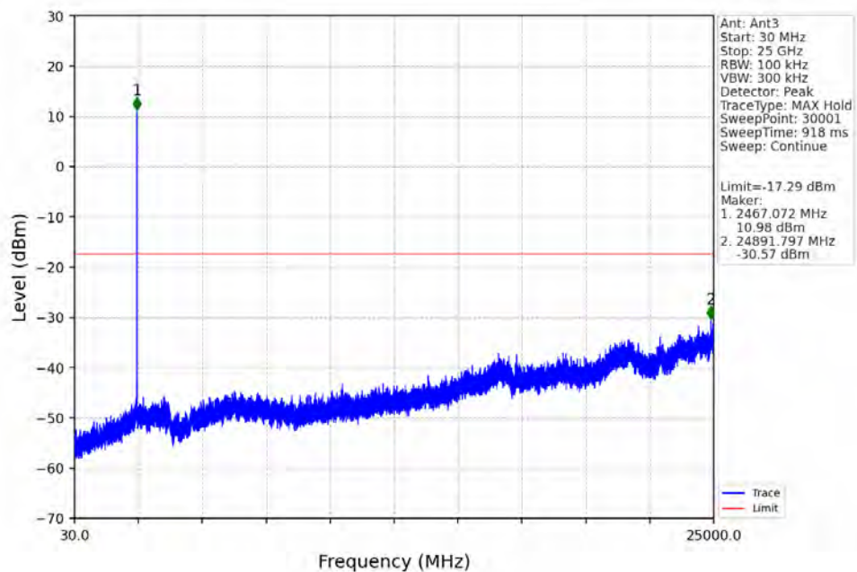
3M_HCH_2468.2MHz_Ant3_NTNV
