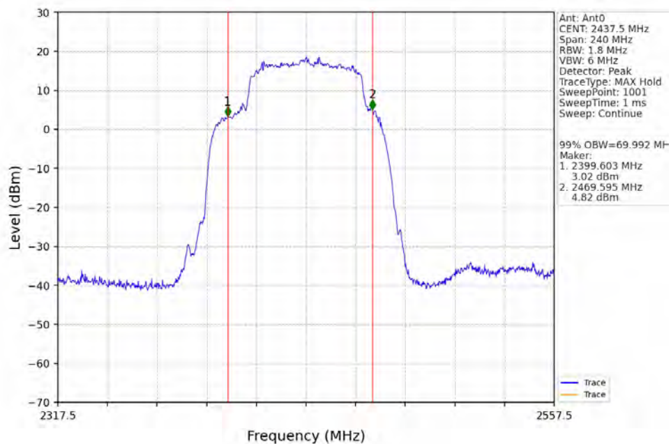
60M_MCH_2437.5MHz_Ant0_NTNV
