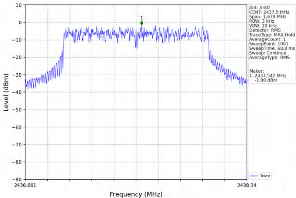
1.4M_MCH_2437.5MHz_Ant0_NTNV
