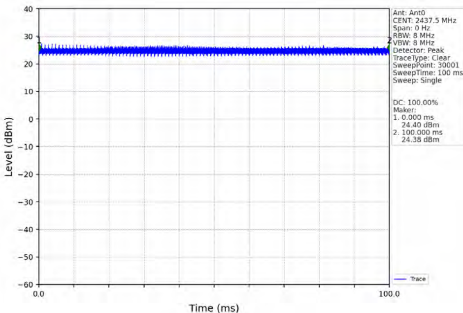
20M_MCH_2437.5MHz_Ant0_NTNV
