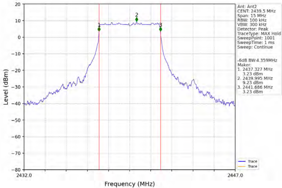
5M_MCH_2439.5MHz_Ant2_NTNV
