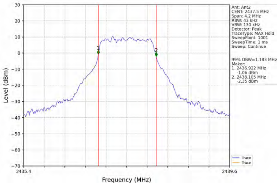
1.4M_MCH_2437.5MHz_Ant2_NTNV
