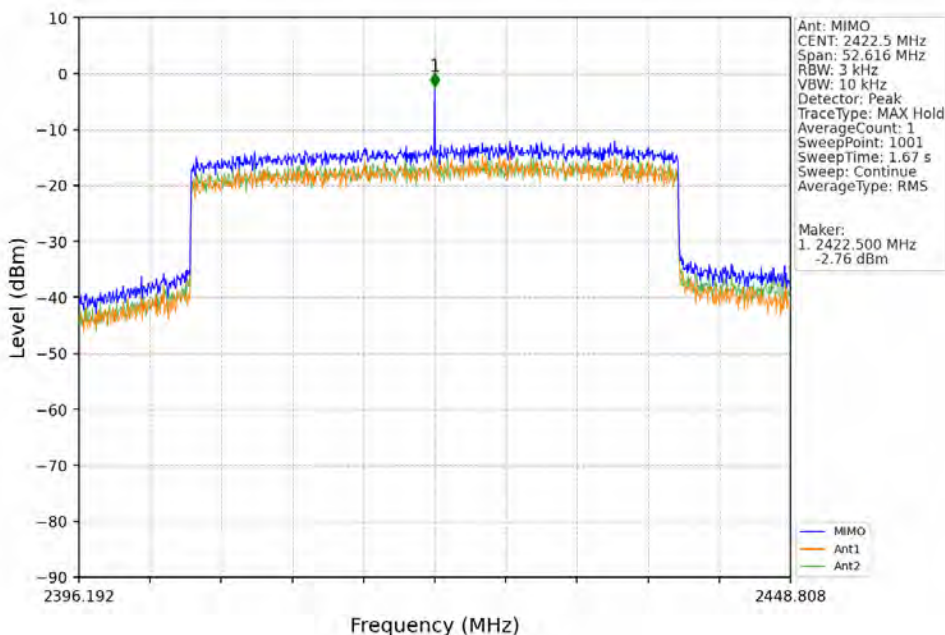
40M_LCH_2422.5MHz_MIMO_NTNV
