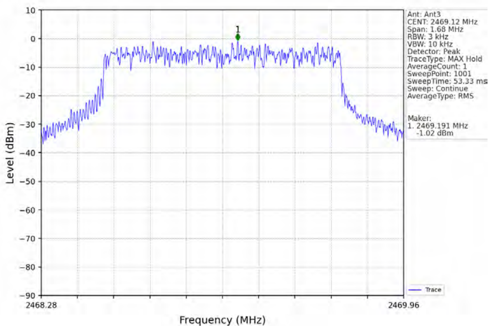
1.4M_HCH_2469.12MHz_Ant3_NTNV
