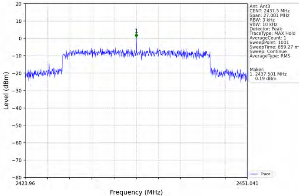
20M_MCH_2437.5MHz_MIMO_NTNV
