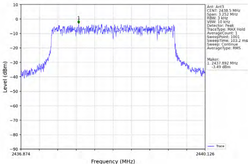
3M_MCH_2438.5MHz_Ant3_NTNV
