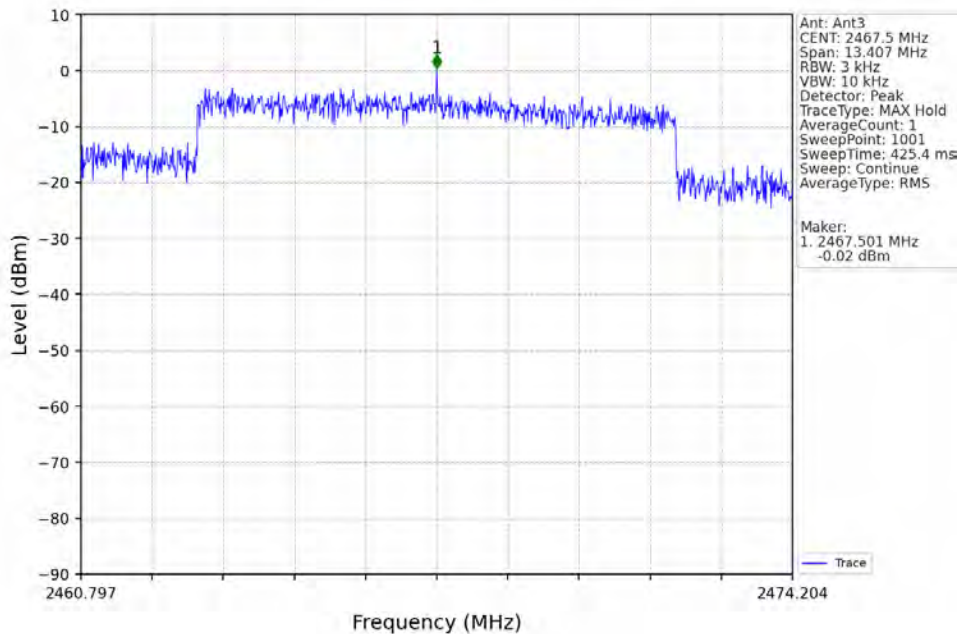
10M_HCH_2467.5MHz_MIMO_NTNV
