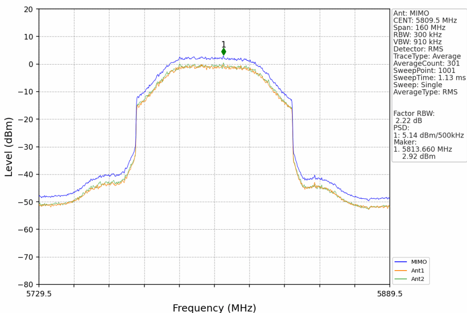
80M_HCH_5809.5MHz_MIMO_NTNV
