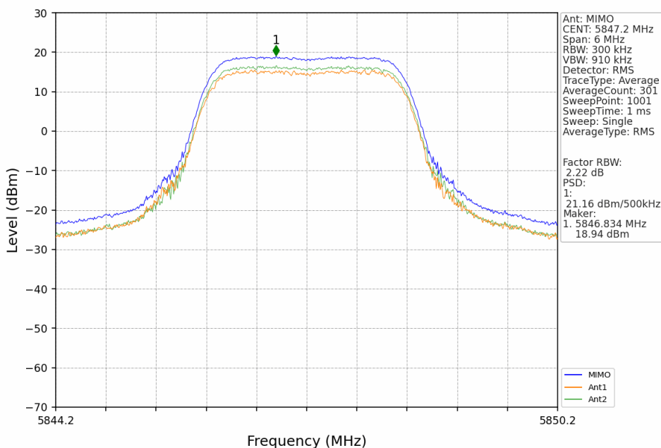
3M_HCH_5847.2MHz_MIMO_NTNV
