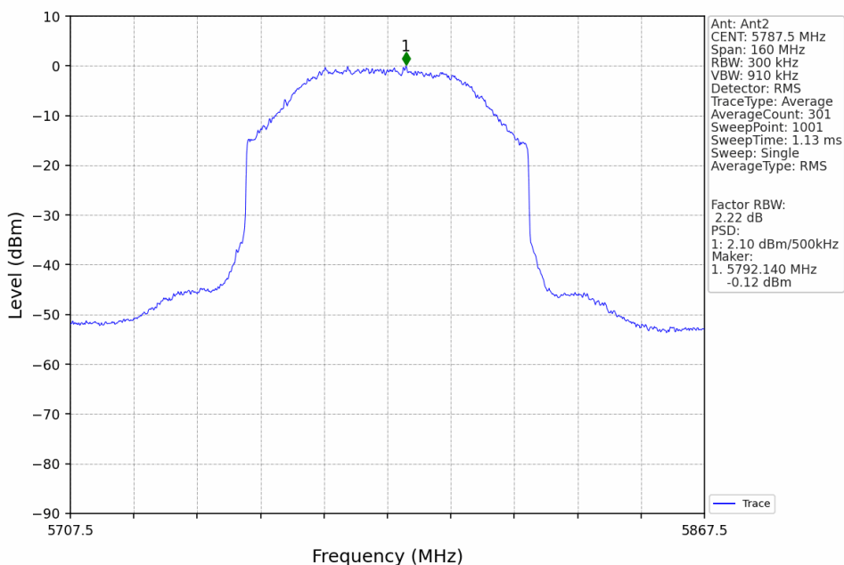
80M_MCH_5787.5MHz_Ant2_NTNV
