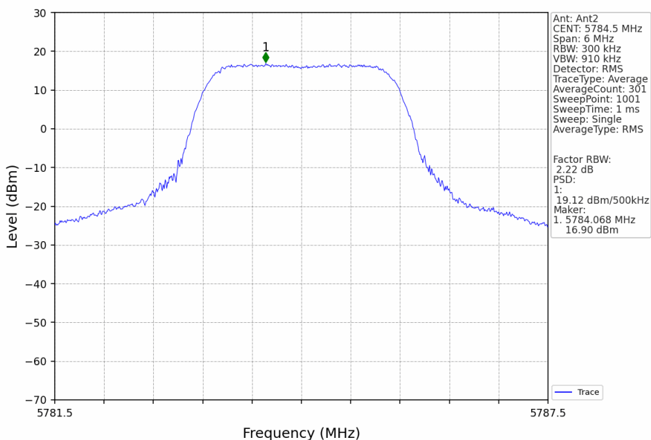
3M_MCH_5784.5MHz_Ant2_NTNV
