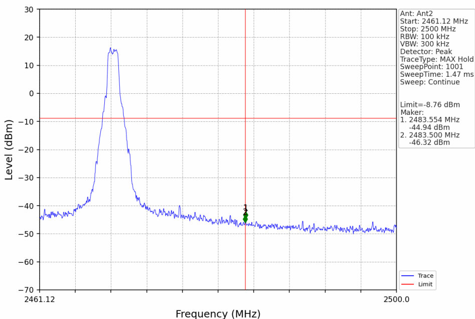
1.4M_HCH_2469.12MHz_Ant2_NTNV
