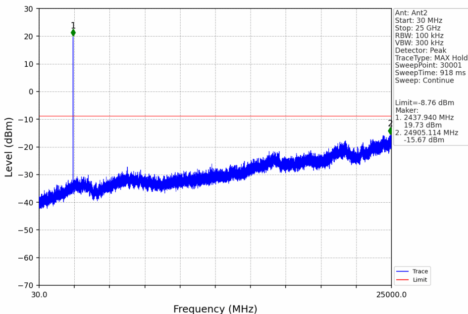
1.4M_MCH_2437.5MHz_Ant2_NTNV
