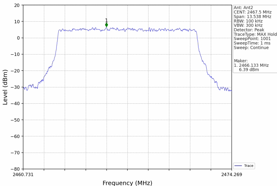
10M_HCH_2467.5MHz_Ant2_NTNV
