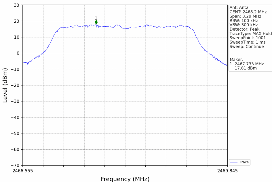
3M_HCH_2468.2MHz_Ant2_NTNV
