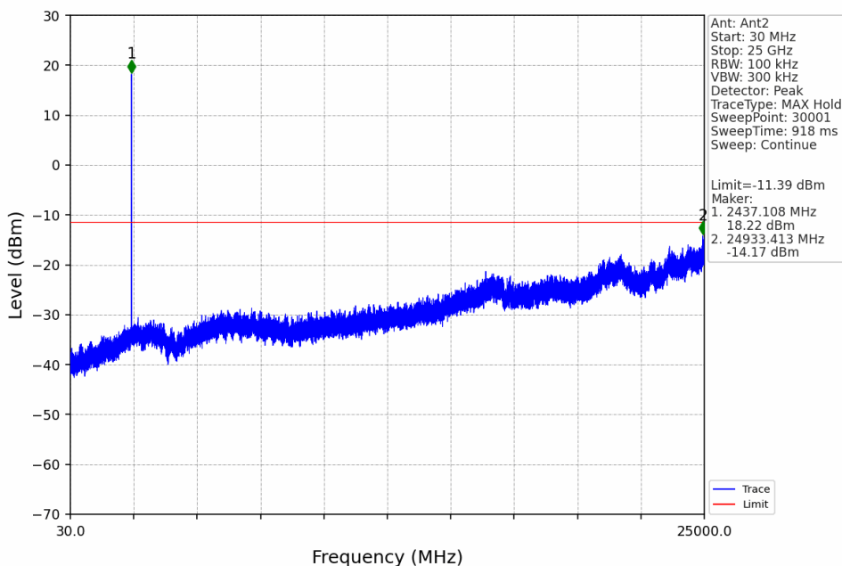
5M_MCH_2437.74MHz_Ant2_NTNV
