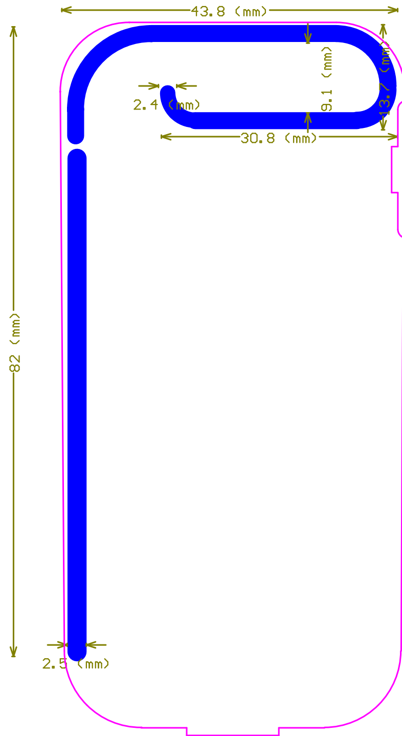
天线尺寸图
