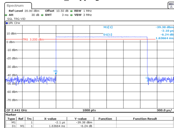
DH3_Hopping 1.637ms
