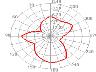
2450.000MHz E1
