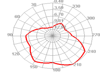
2450.000MHz E2
