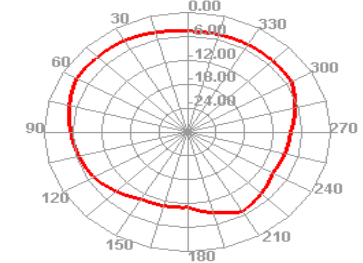
2450.000MHz H
