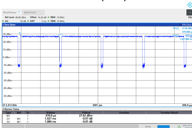
802.11ax(HE20)
