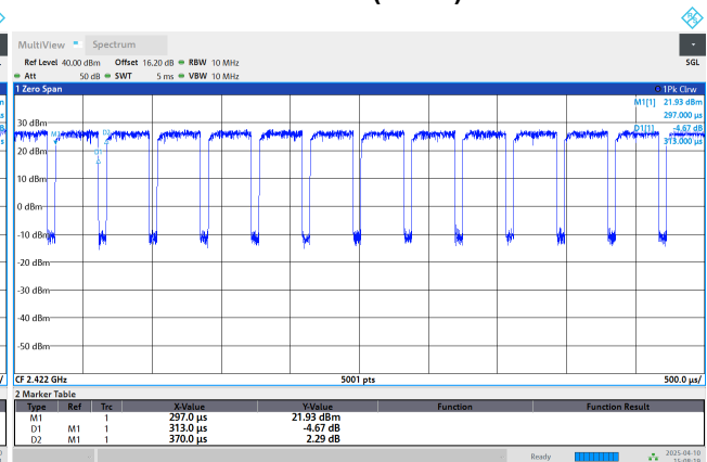
802.11ax(HE40)
