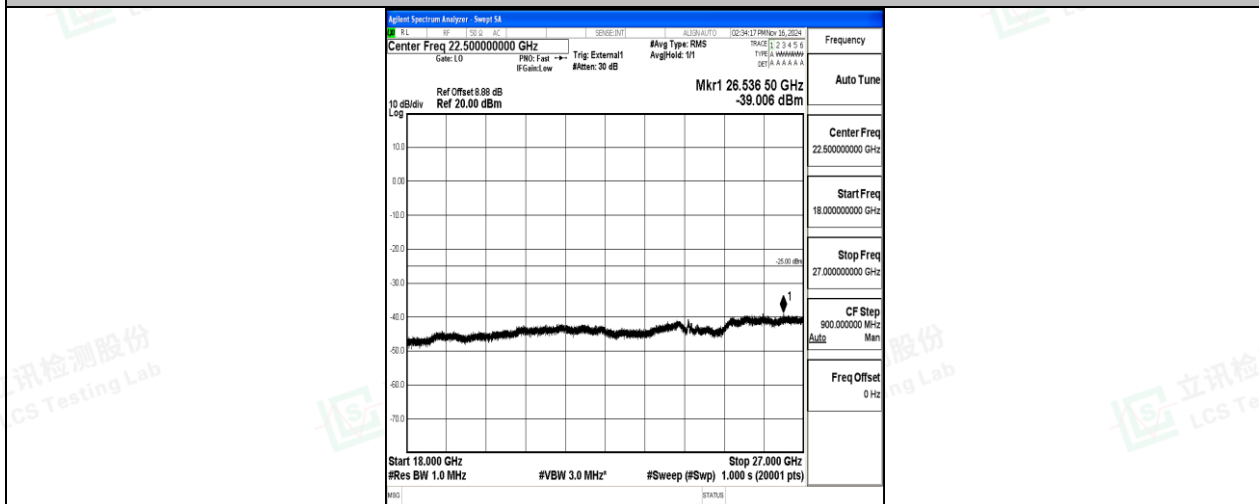
Band41-20MHz-16QAM-41490-1RB#0-18000~27000-PASS
