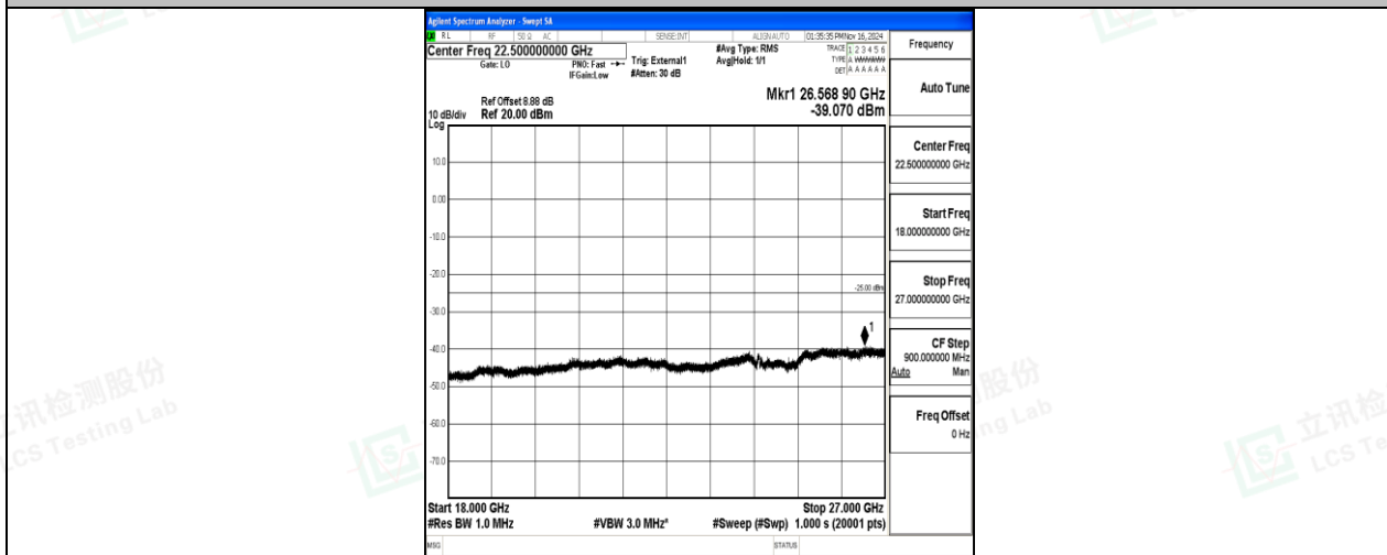
Band41-15MHz-QPSK-39725-1RB#0-18000~27000-PASS
