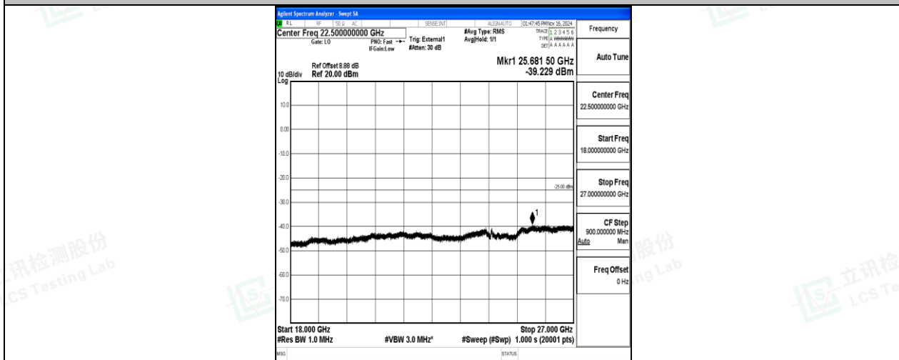
Band41-15MHz-16QAM-41515-1RB#0-18000~27000-PASS
