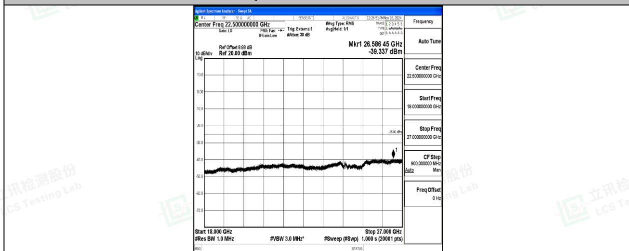
Band41-5MHz-QPSK-41565-1RB#0-18000~27000-PASS
