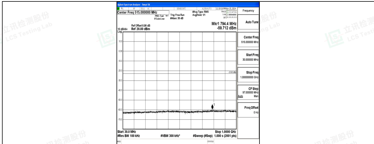
Band2-20MHz-QPSK-18700-1RB#0-30~1000-PASS
