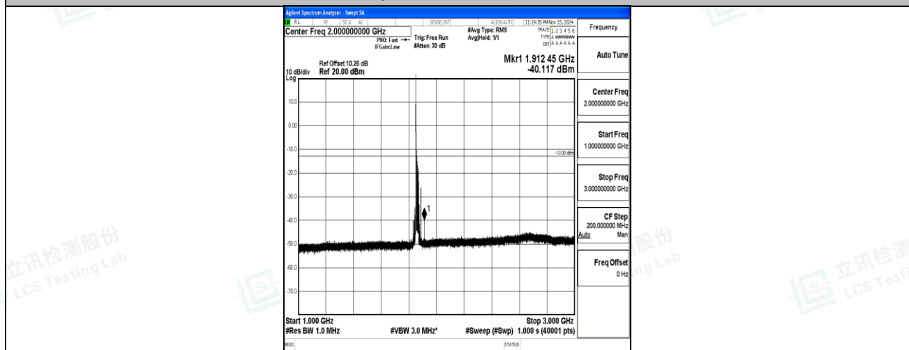
Band2-20MHz-QPSK-18700-1RB#0-1000~3000-PASS
