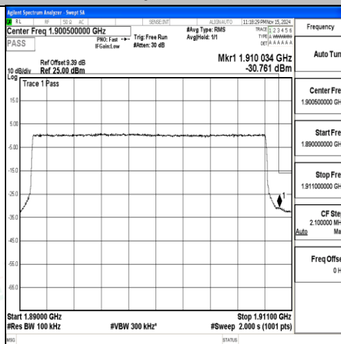
Band2-20MHz-OPSK-19100-100RB#0-PASS
